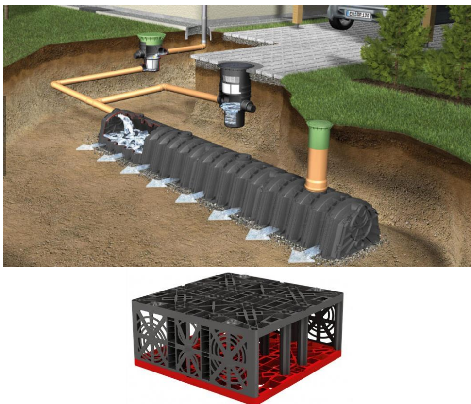
Obr. 5.16 Akumulačná nádrž s priepadom do vsakovacieho objektu (tunel, resp. kôš)
