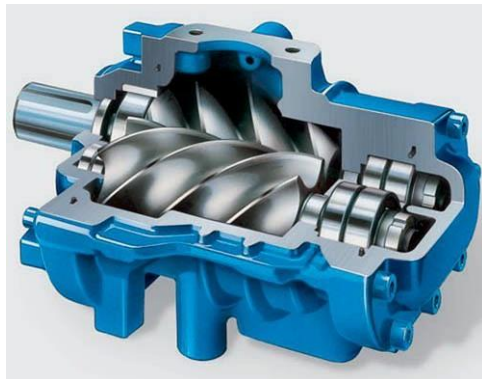
Obr. 2.6 Skrutkový kompresor
