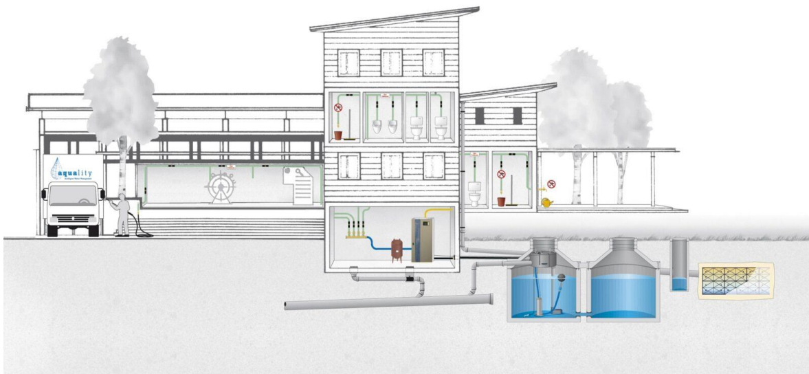
Obr. 5.12 Systémy využitia zrážkovej vody v administratívnej budove
