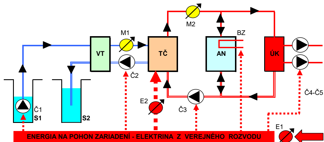
Obr. 6.63 Schéma zapojenia tepelného čerpadla voda/voda v systéme výroby tepla pre vykurovanie v bivalentnom zapojení
