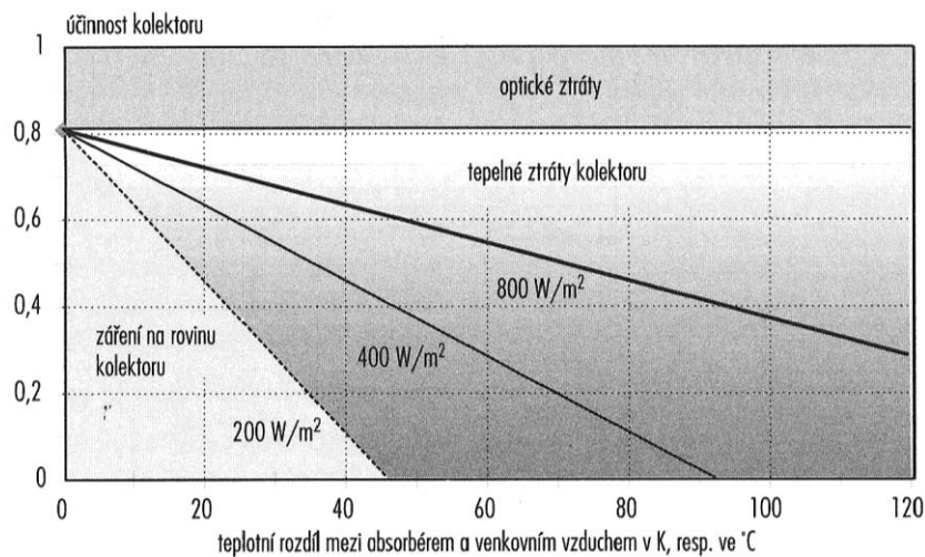
Obr. 6.24 Účinnosť kolektora ako funkcia rozdielu teplôt medzi absorbérom a okolím pri slnečnom žiarení 800, 400 a 200 \text{W}/\text{m}^2 .
