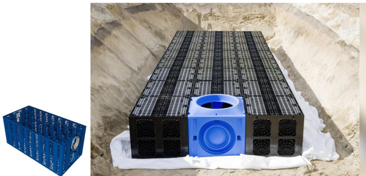
Obr. 5.27 Vsakovacie bloky
