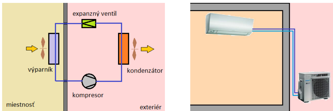
Obr. 2.15 Priame kompresorové chladenie
