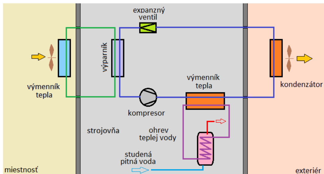
Obr. 2.22 Schéma nepriameho kompresorového chladenia
