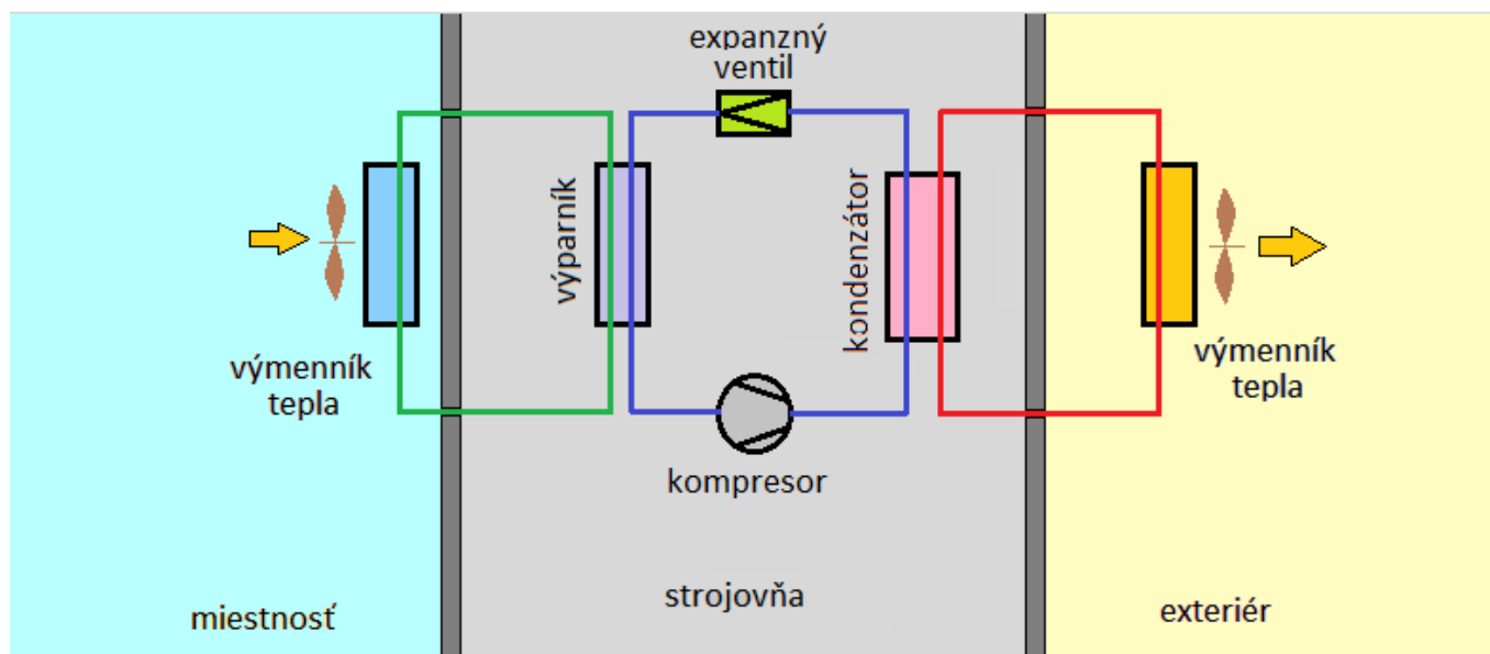
Obr. 2.20 Schéma nepriameho kompresorového chladenia
