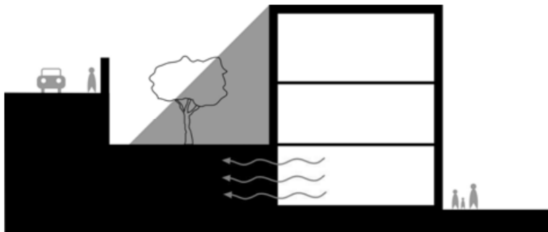
Obr. 2.28 Prenos tepla medzi vnútorným prostredím a pôdou
