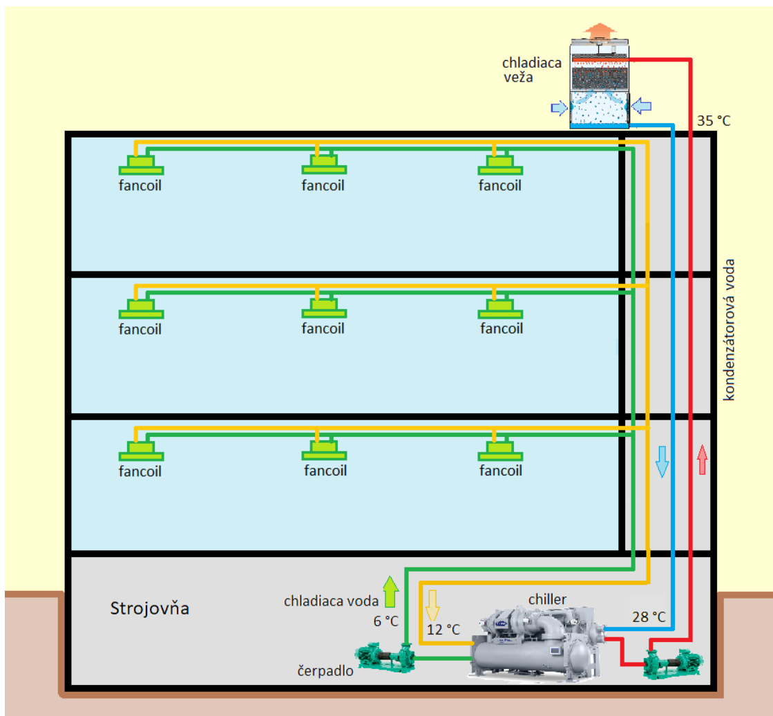
Obr. 2.21 Schéma nepriameho kompresorového chladenia v administratívnej budove
