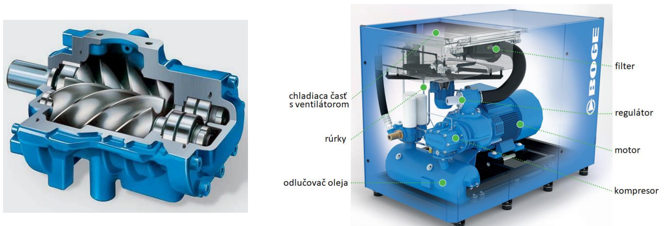
Obr. 2.6 Skrutkový kompresor
