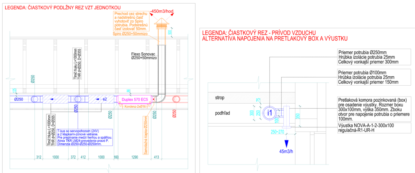
Obr. 2.62 Detail a čiastkový rez VZT potrubím a pretlakovou komorou s výustkou – popis komponentov a detail
