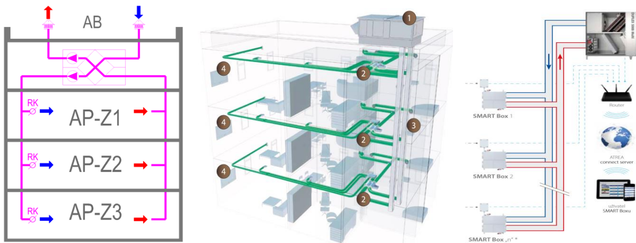
Obr. 2.32 Aplikácia inteligentného systému vetrania DCV po jednotlivých podlažiach v administratívnej budove (AB) – centrálna jednotka
