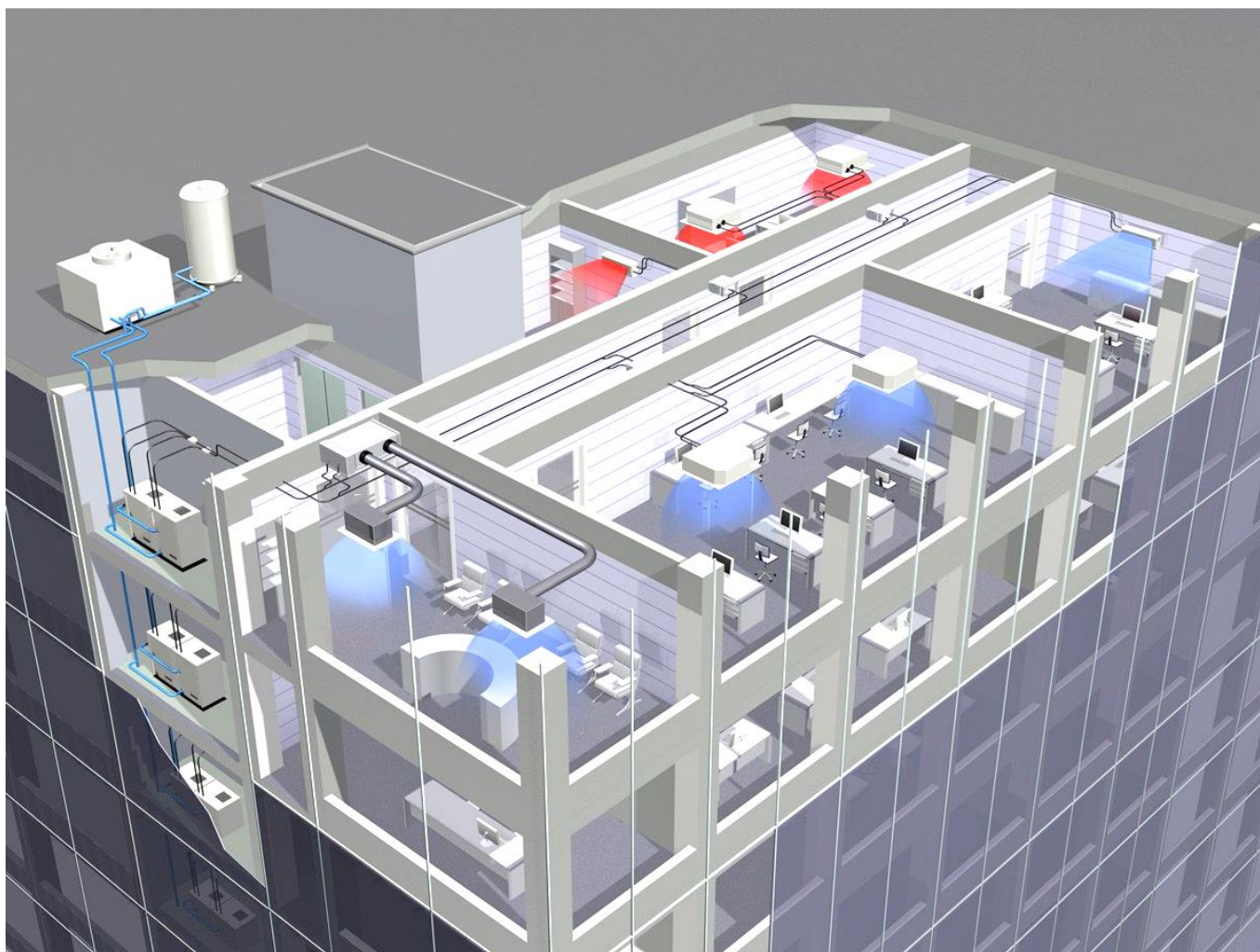
Obr. 2.19 VRV systém so spätným získavaním tepla vodný (Daikin)
