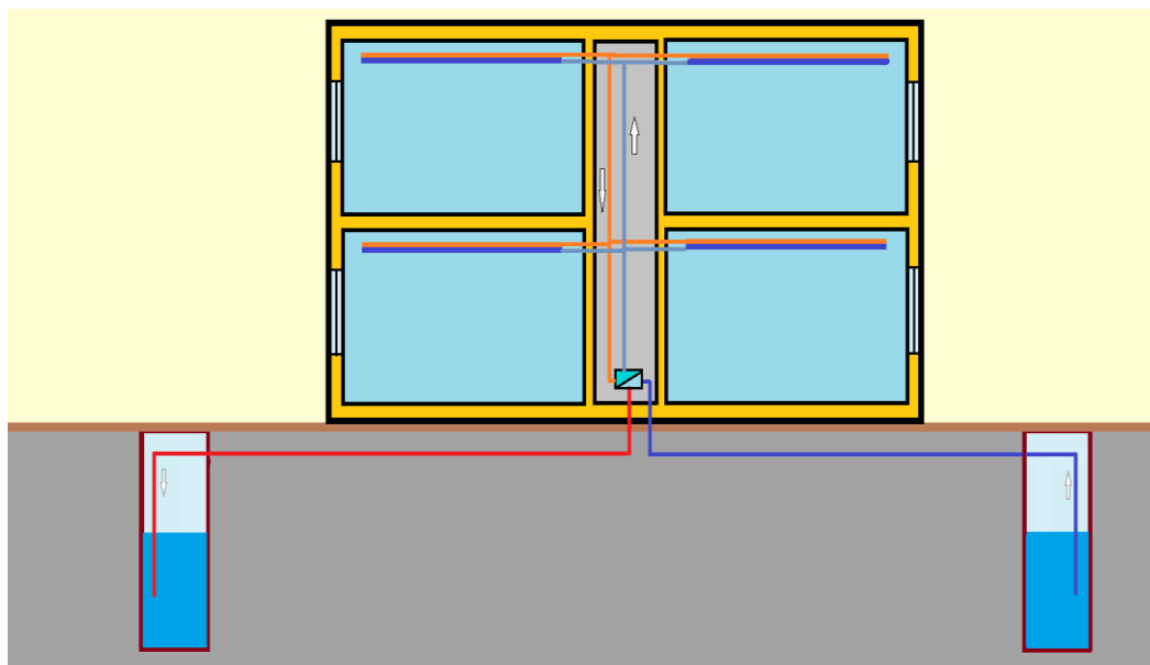
Obr. 2.25 Nepriame chladenie studňovou vodou
