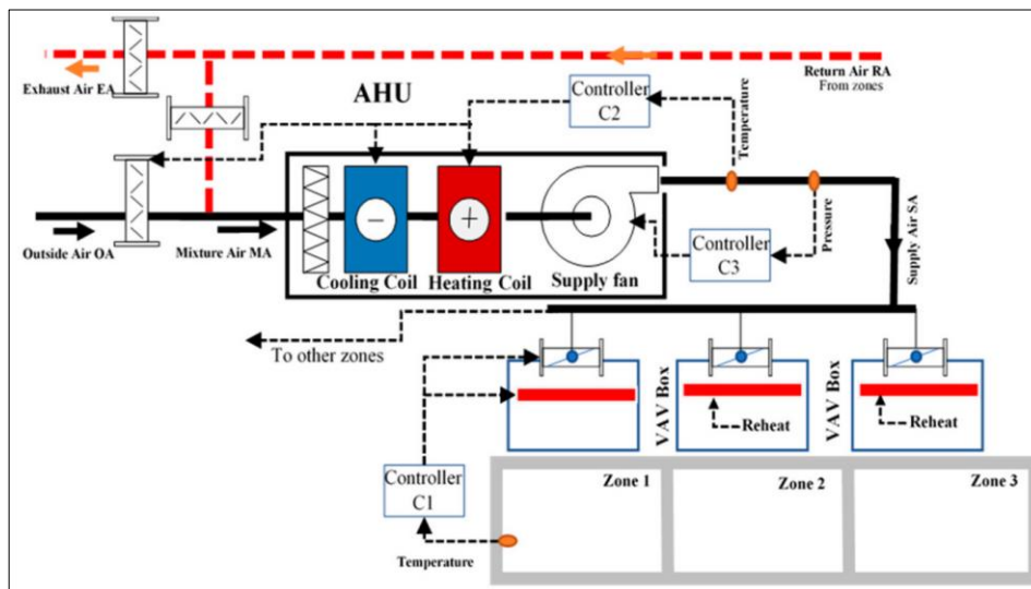
Obr. 2.37 Procesná schéma systému vetrania - vetrací systém VAV
