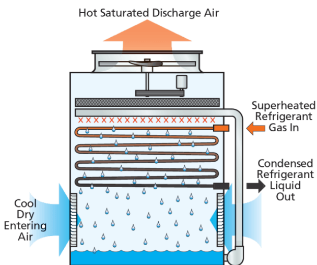
Obr. 2.13 Odparovací kondenzátor
