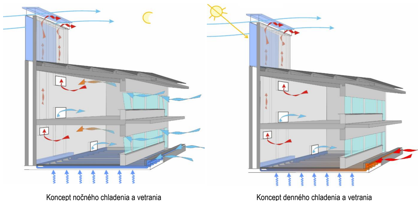
Obr. 2.24 Chladenie zabezpečené nočným prirodzeným vetraním
