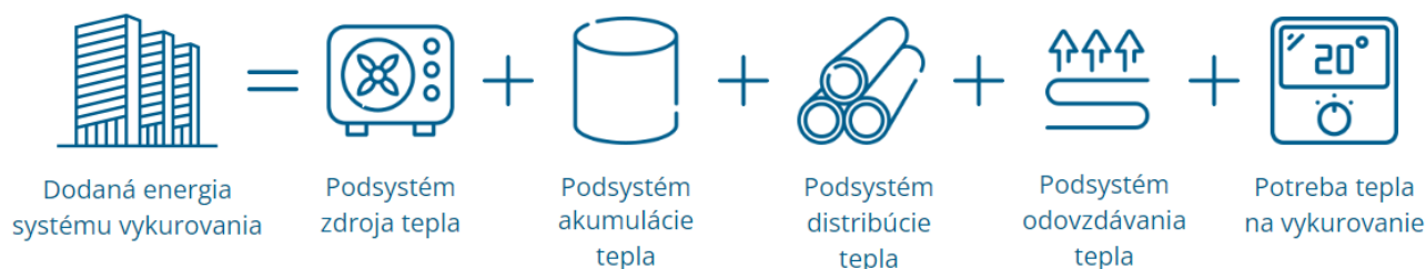
Obr. 4.27 Grafické znázornenie postupu pre stanovenie dodanej energie systému vykurovania
