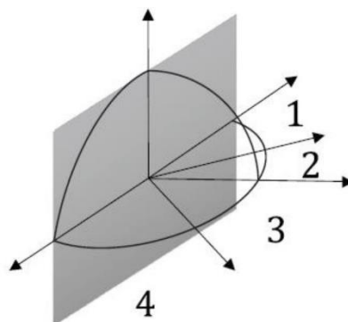
Obr. 4.15 Mesačné výpočtové postupy: rozdelenie oblohy do 8 segmentov, so 4 segmentami vzhľadom na tienový objekt
