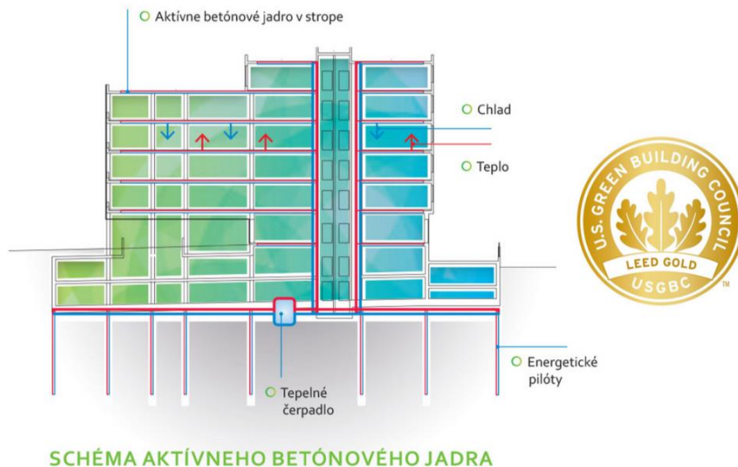
Obr. 4.3 Administratívne budovy – EcoPoint schematický rez objektom
