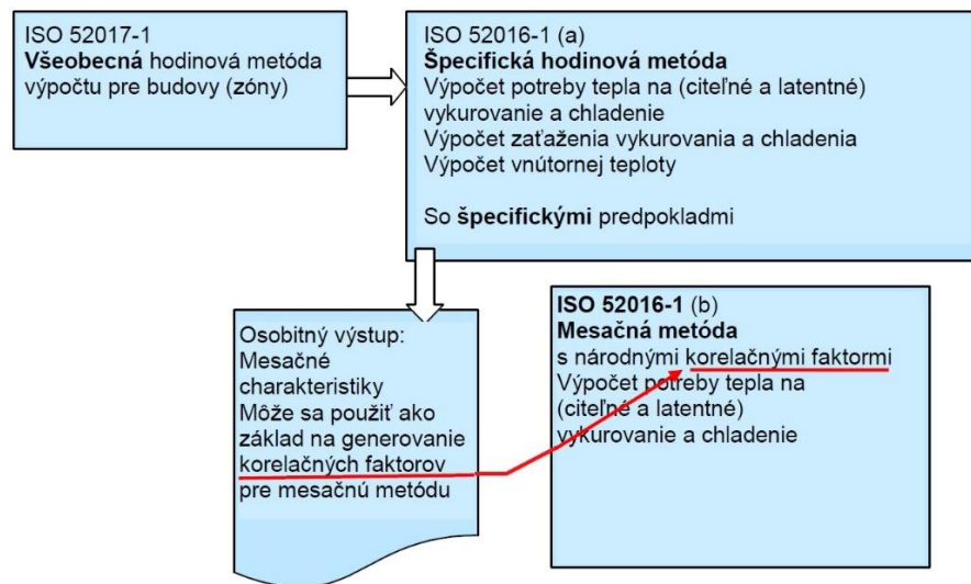
Obr. 4.11 Vzťah medzi ISO 52016-1 a ISO 52017-1
