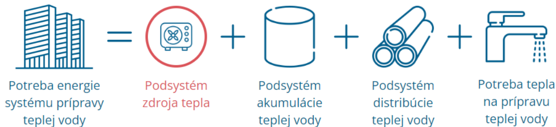
Obr. 4.17 Grafické znázornenie postupu pre stanovenie potreby energie systému prípravy teplej vody
