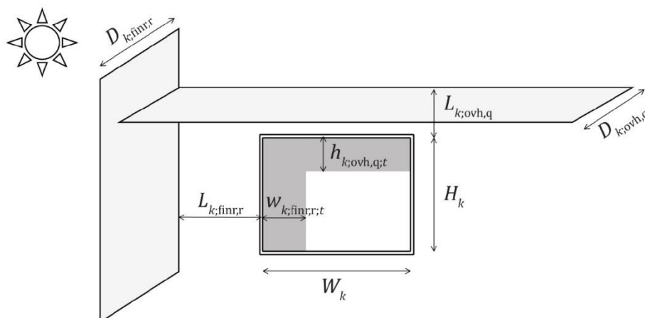
Obr. 4.13 Geometria jednoduchých vystupujúcich konštrukcií alebo bočných stien
