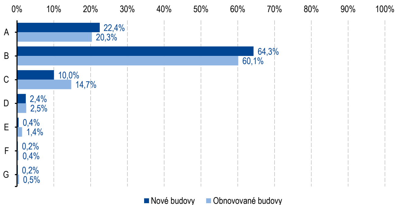
Obr. 4.6 Podiel energetických tried administratívnych budov na Slovensku za obdobie rokov 2016 - 2021
