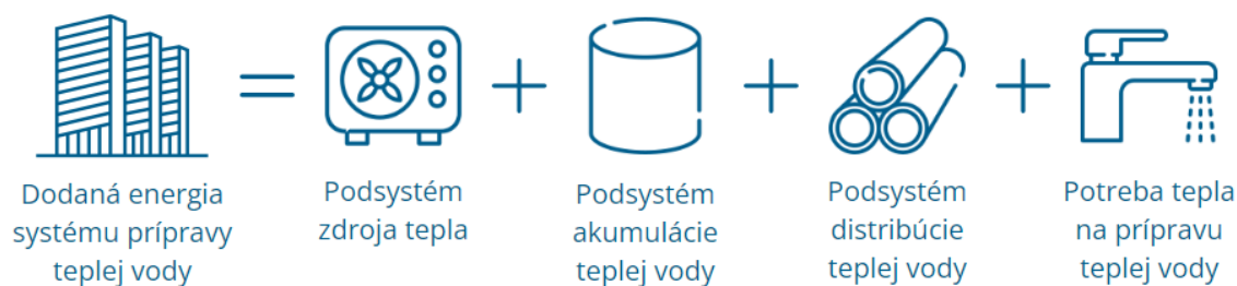
Obr. 4.18 Grafické znázornenie postupu pre stanovenie dodanej energie systému prípravy teplej vody
